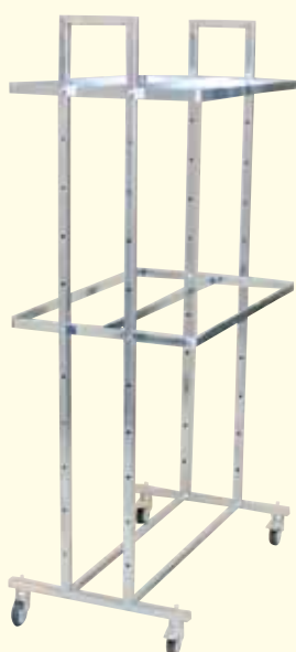
Gateselger L5 M/ 2 dobbelttoppheng. 90 x 55 x H170 cm. Varenr.: 4186-61
